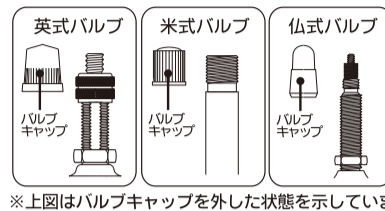
※上図はバルブキャップを外した状態を示しています。
